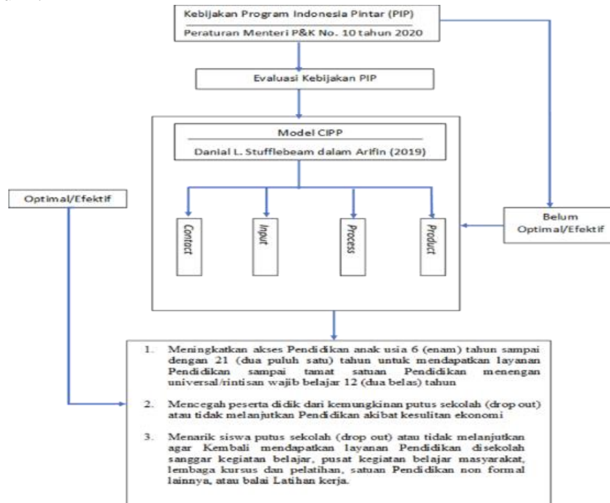
Gambar 1. Kerangka Teori
