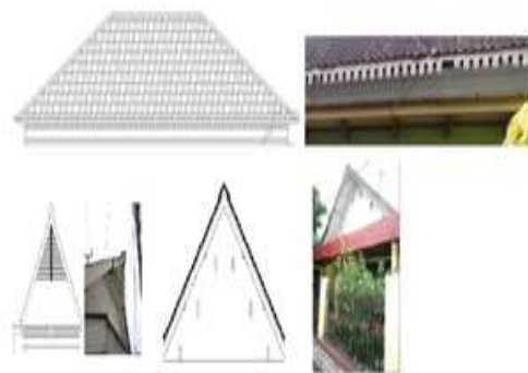
Gambar 4. 8. Bentuk Akhiran Atap Rumah Tinggal Kolonial di Kauman
